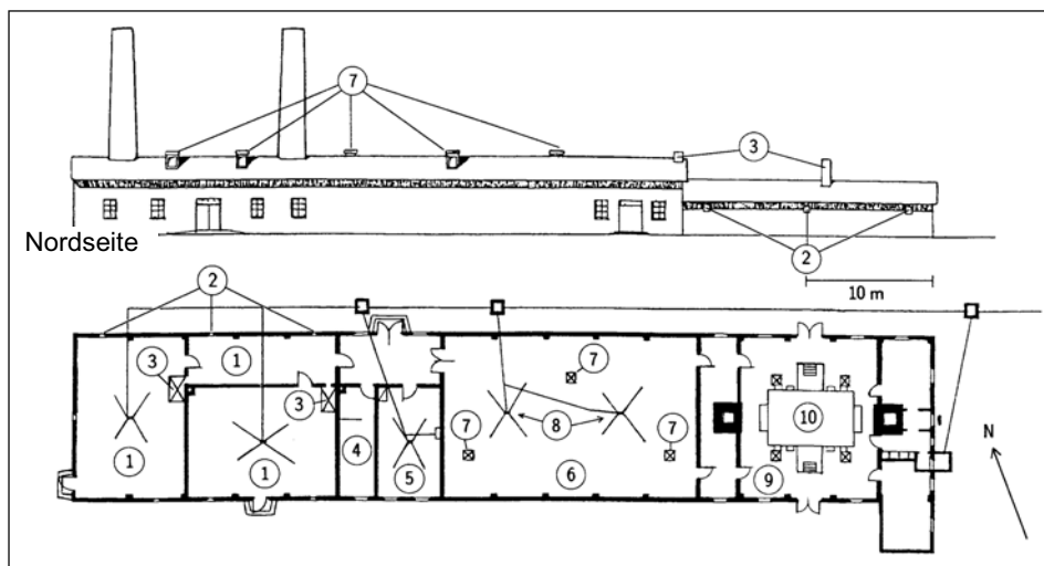
Abbildung 11: Nordseitenansicht (oben) und Grundriß (unten) von Krematorium IV bzw. V (spiegelbildlich) im Lager Auschwitz II/Birkenau. 67
