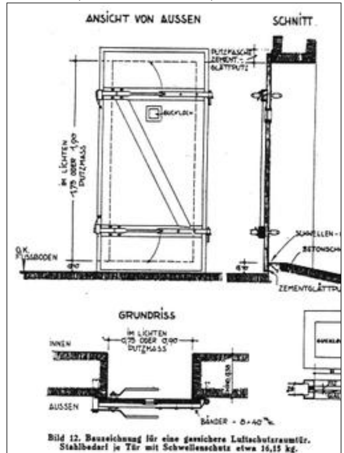
Abbildung 5: Zeichnung einer »gassicheren Luftschutzraumtür«.
