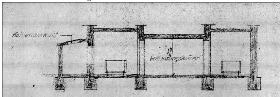
Dokument 2: Querschnitt durch geplante Heißluftentwesungsanlage im KL Majdanek – vgl. “Kohleneinwurf” zur Linken.
